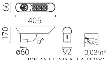
ISKRA LED P ALFA PROG na przejścia dla pieszych dla dróg z ruchem lewostronnym
